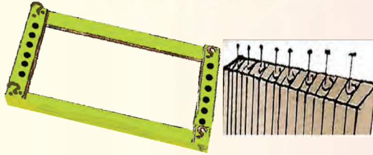
الشكل (١٥٩): طريقة تثبيت المسامير على أضلاع النول.
